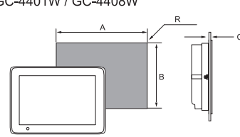
面板开孔尺寸: GC-4401W / GC-4408W
